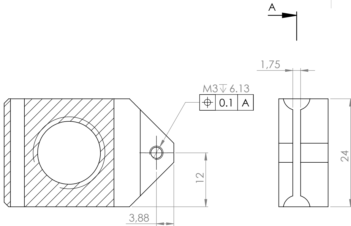
COUPE A-A
