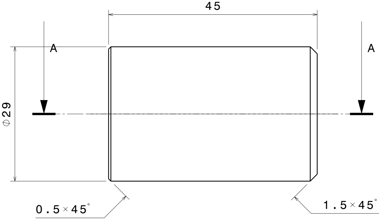
Coupe A-A Echelle : 2:1
