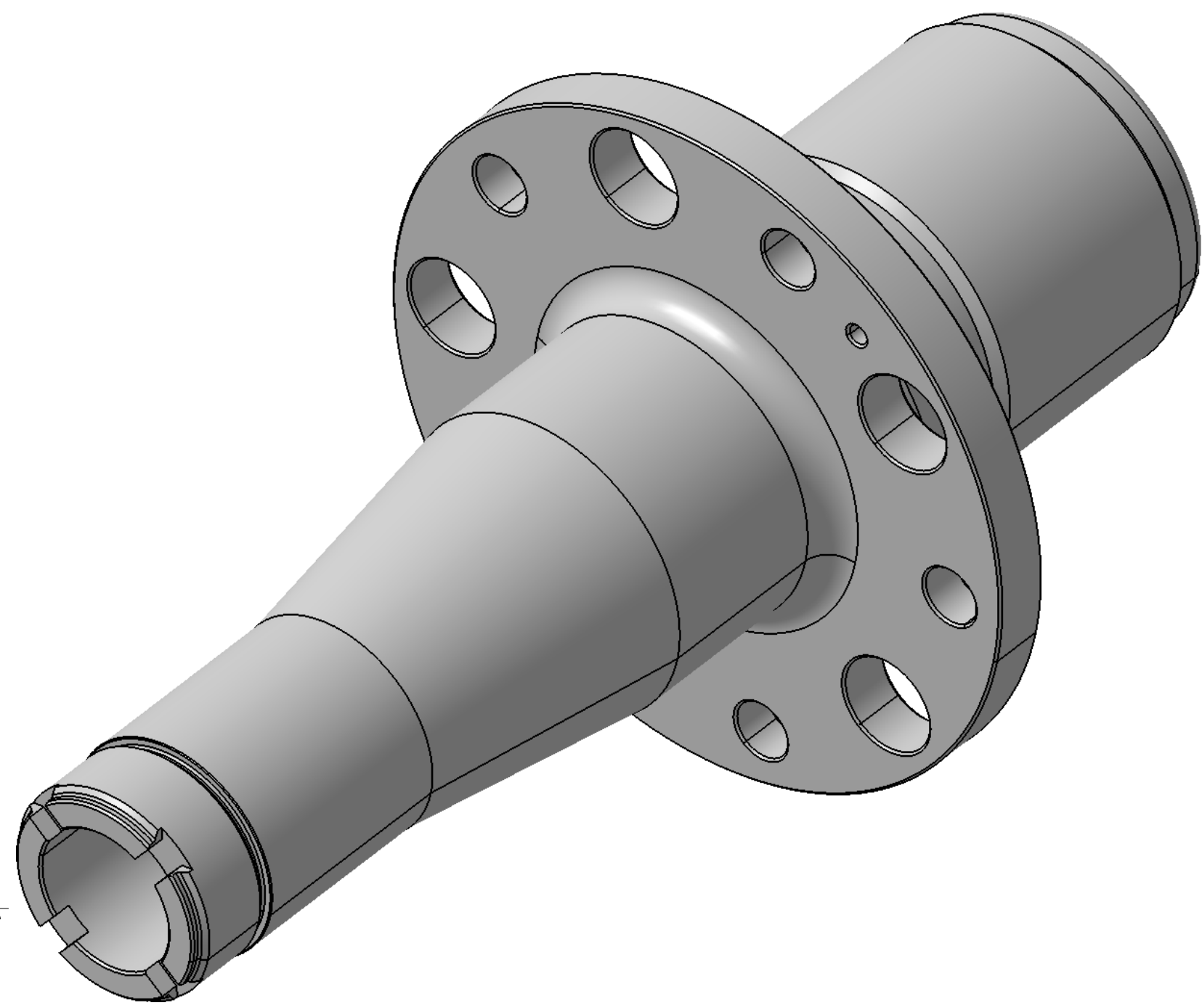
Vue isométrique Echelle : 1:1
