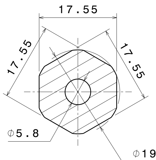
Coupe A-A Echelle : 2:1
