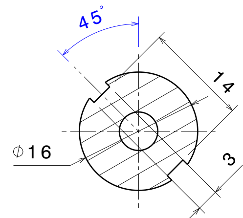
Section D-D Echelle : 2:1
