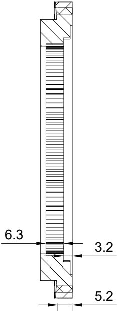
A-A (1:1)
