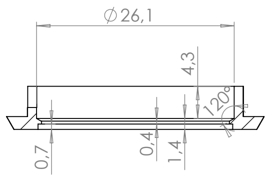
COUPE B-B ECHELLE 2 : 1
