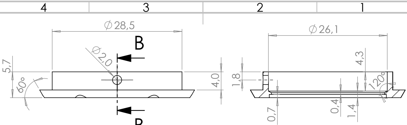
COUPE B-B ECHELLE 2 : 1
