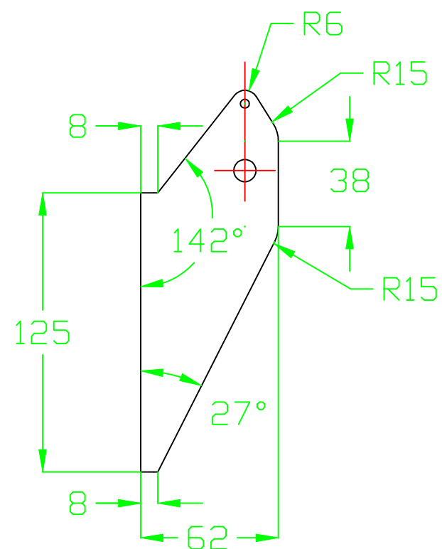
View A-A
