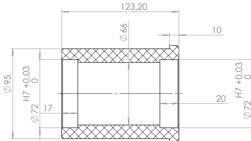
COUPE A-A
