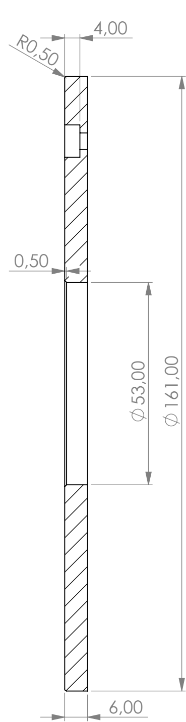
A-A (1 : 1)
