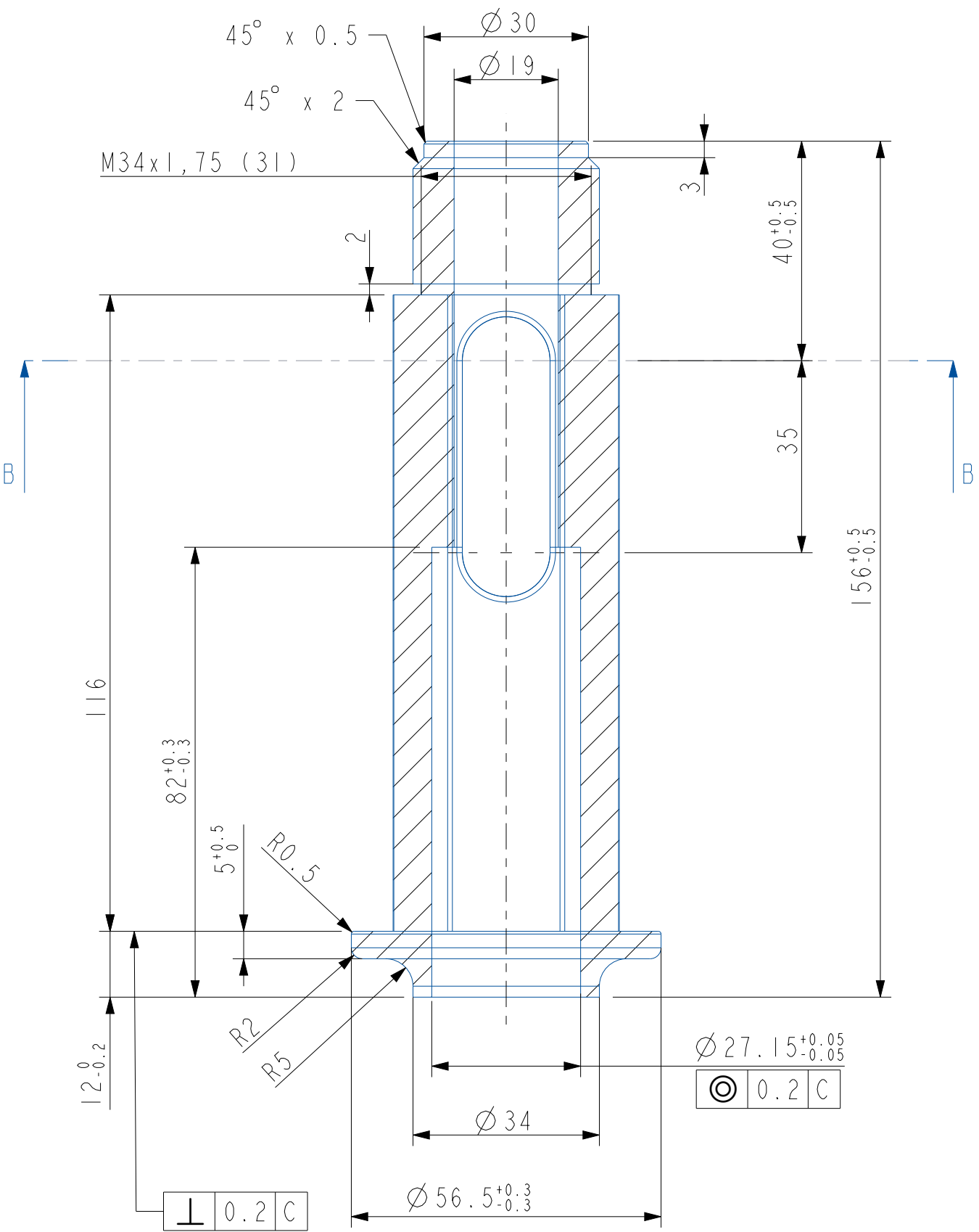
COUPE A-A
