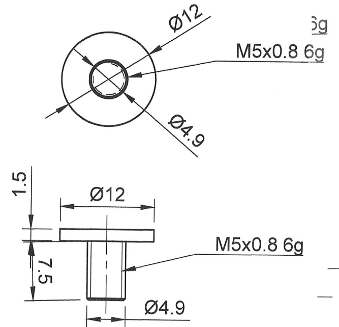
Pièce 2 (Vis)
