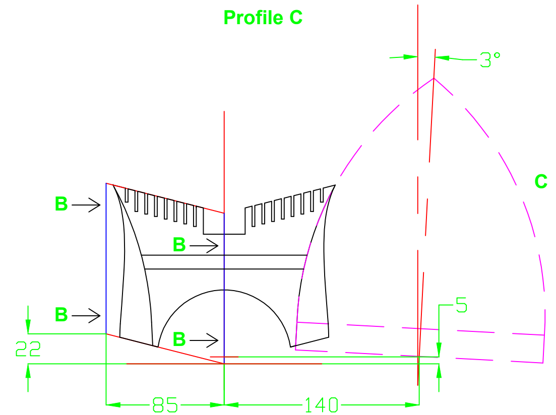
View A-A
