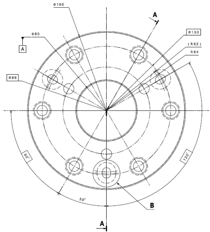
Vue de face Echelle : 1:1
