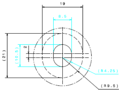
Détail B Echelle : 2:1 3 usinages identiques
