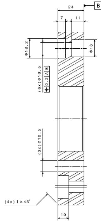
Coupe A-A Echelle : 1:1
