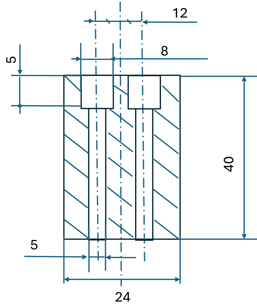
Coupe A-A
