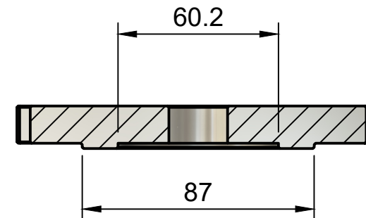
C-C (1:2)
