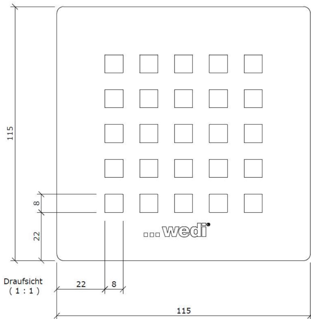
Ansicht ( 1 : 1 )
