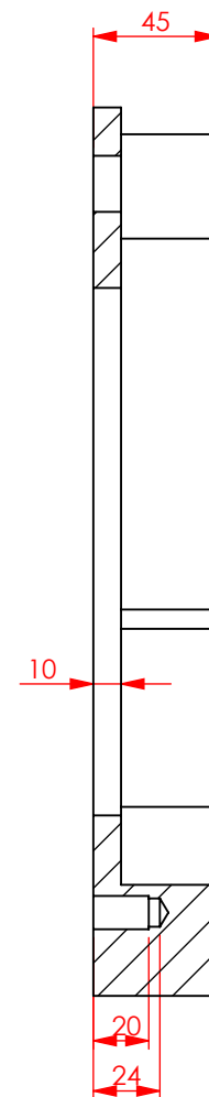
SECTION A-A
