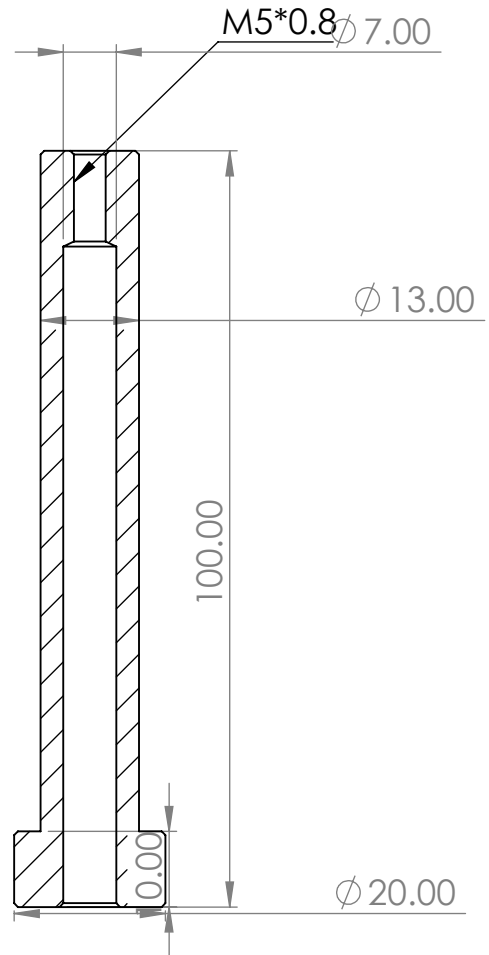
COUPE A-A
