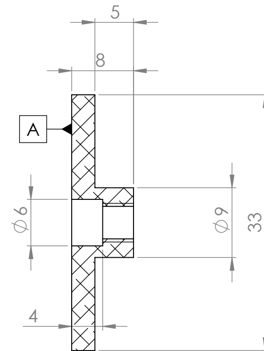
COUPE A-A
