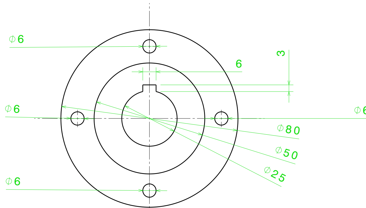
Vue de face Echelle : 1:1
