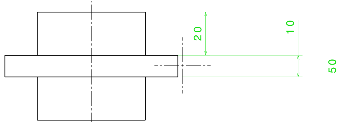
Vue de dessous Echelle : 1:1
