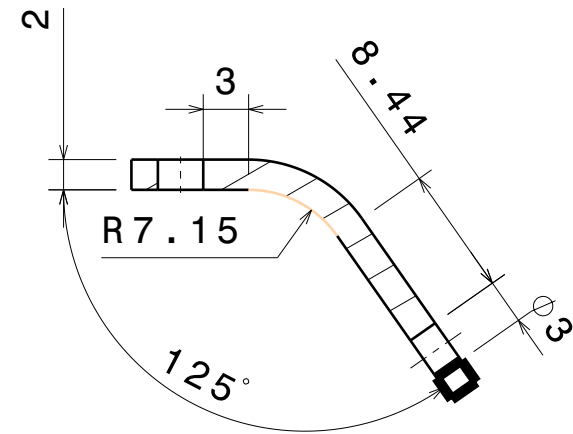
Coupe A-A Echelle : 2:1
