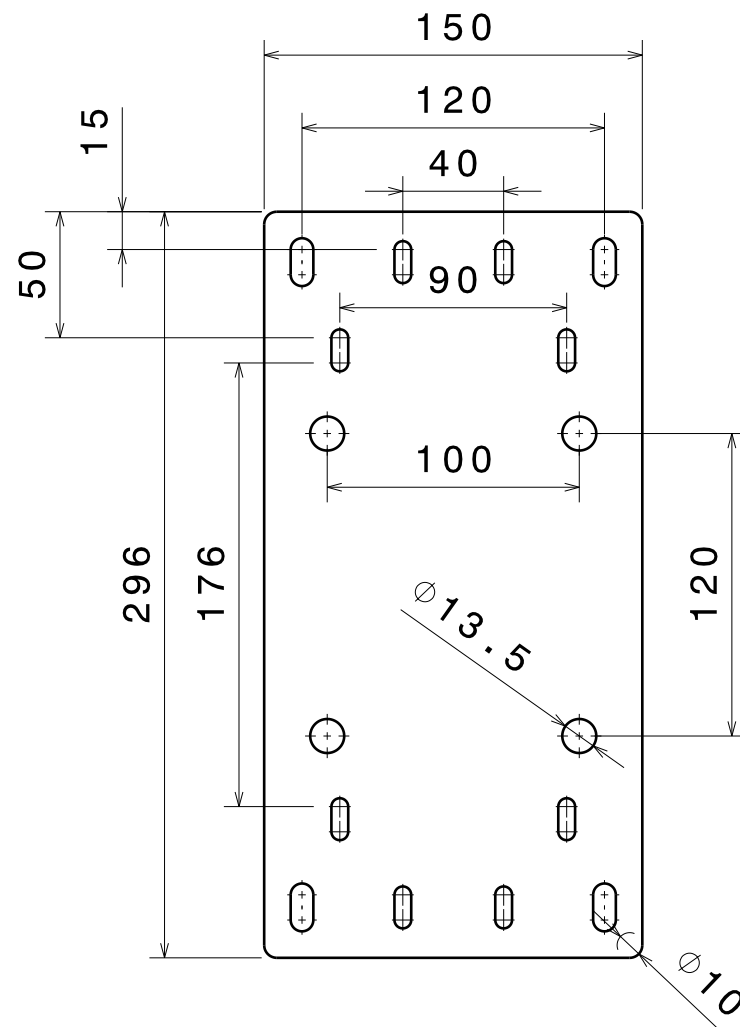
Vue de derrière Echelle : 1:3
