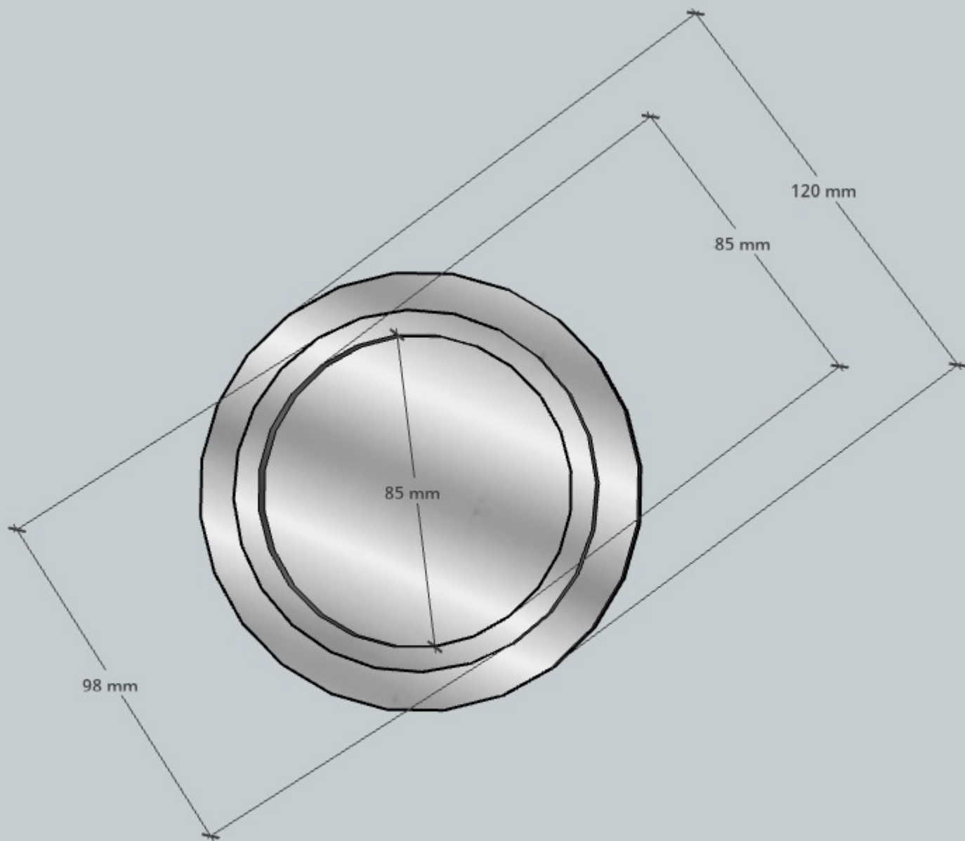
VUE DE DESSOUS MANCHON Ø 120 mm
