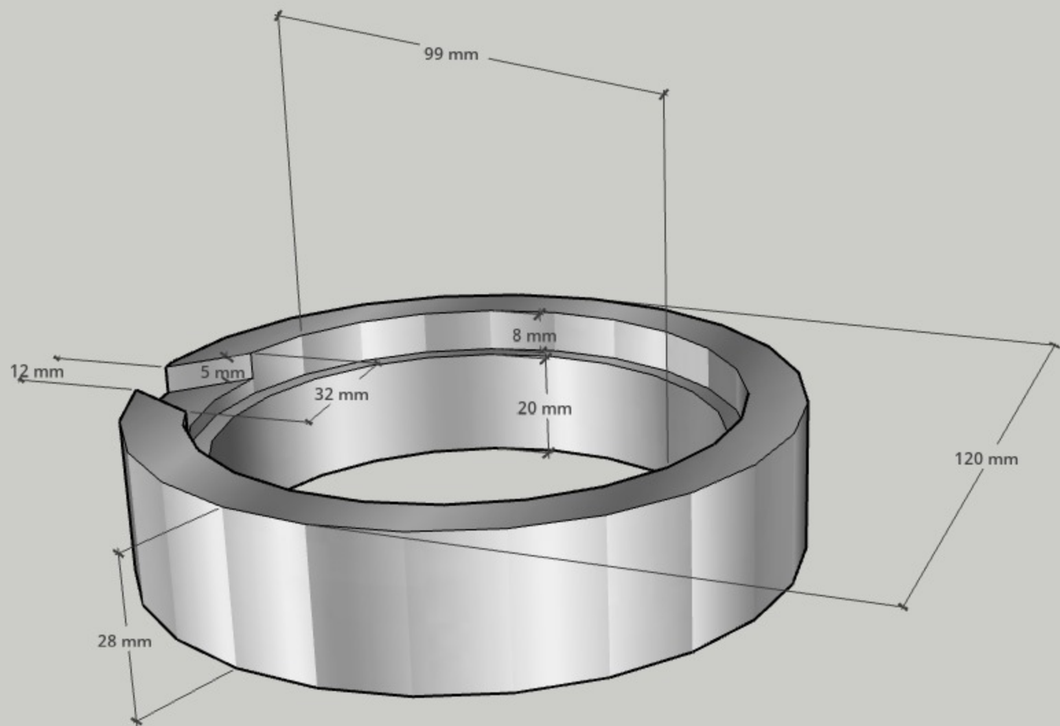
VUE DE COTÉ BAGUE Ø 120 mm
