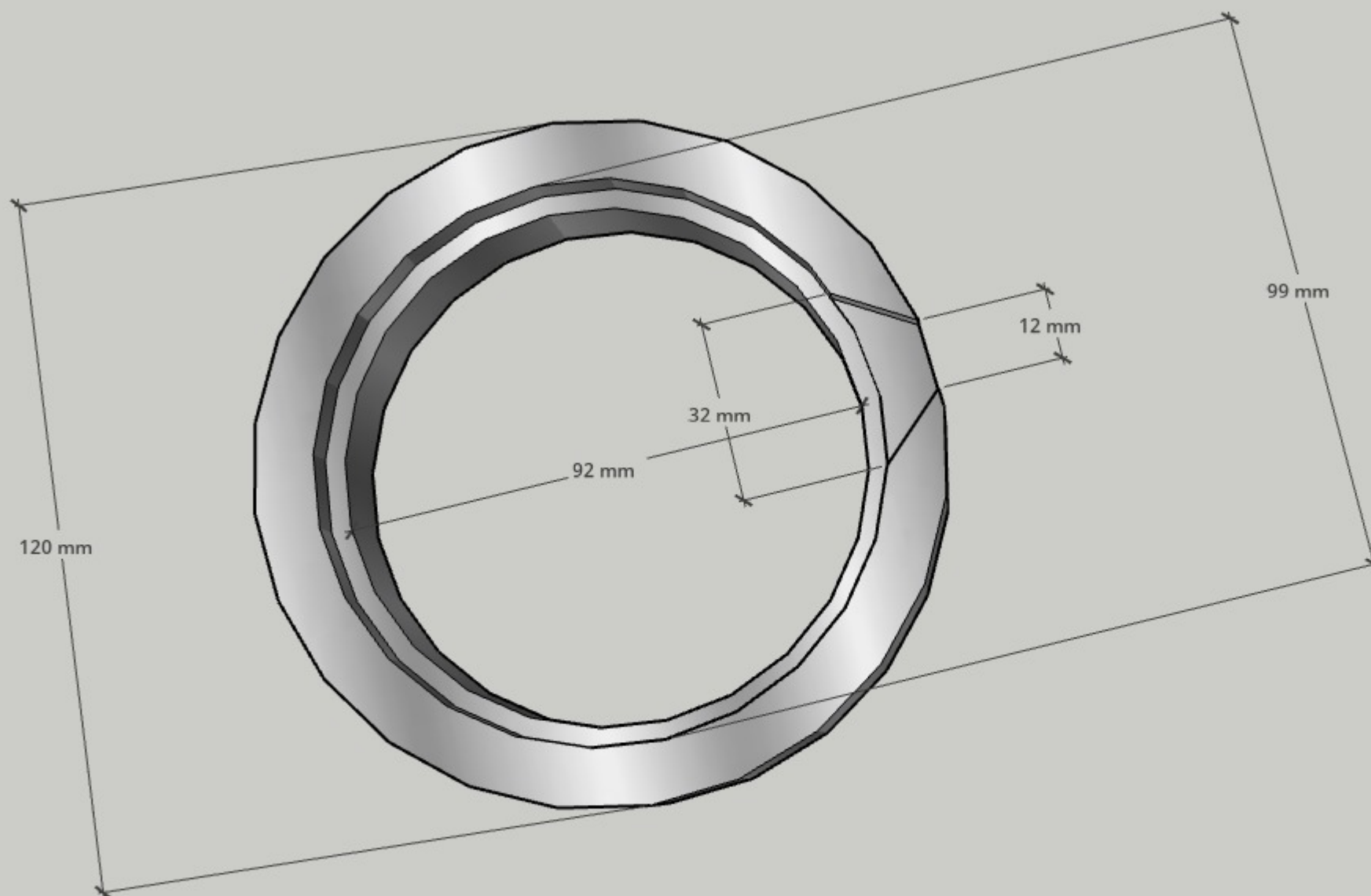
VUE DE DESSUS BAGUE Ø 120 mm
