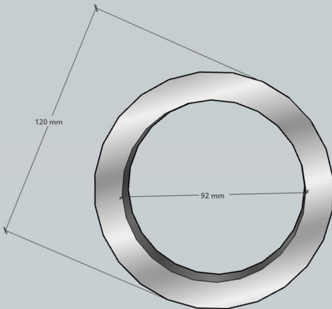
VUE DE DESSOUS BAGUE Ø 120 mm
