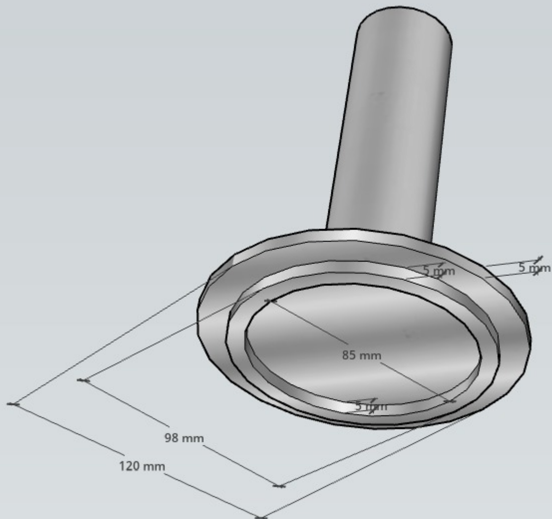
VUE DE DESSOUS 3D MANCHON Ø 120 mm
