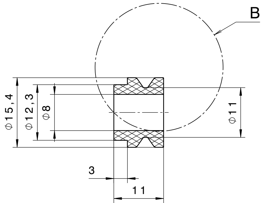
Coupe A-A Echelle : 2:1
