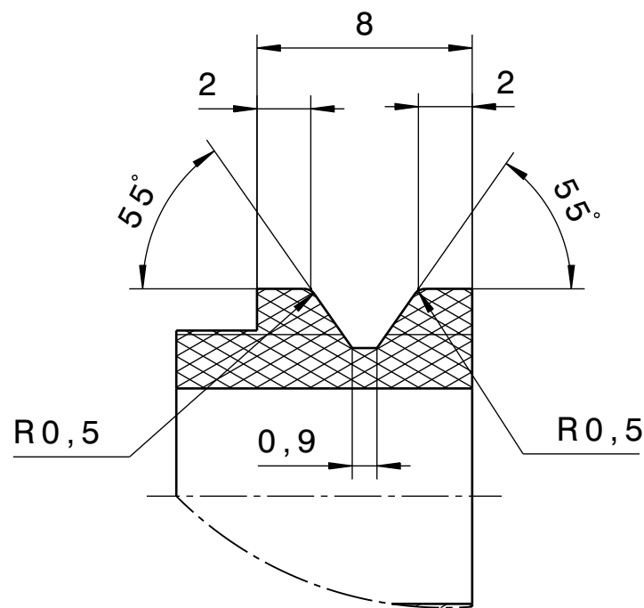
Détail B Echelle : 4:1
