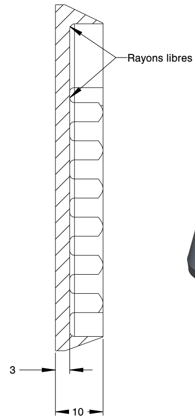
COUPE B-B
