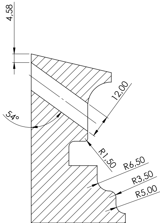
COUPE A-A
