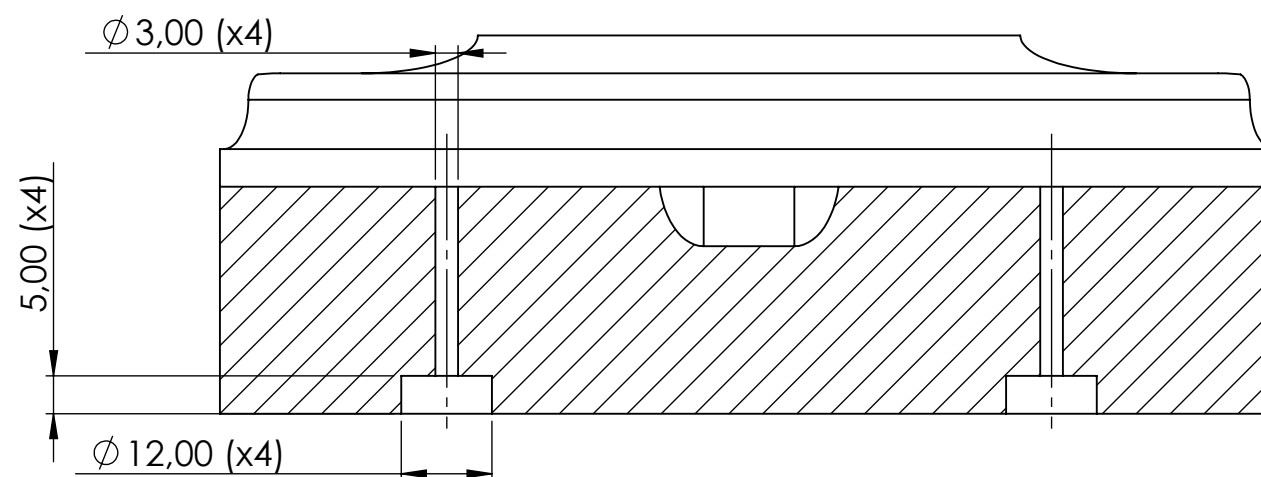
COUPE D-D
