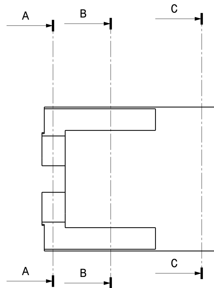
Left view Scale: 1:1
