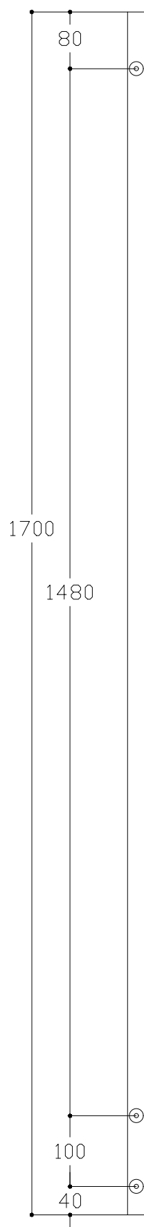
Plan face 1 tube inox longueur 1.70m Percement diamètre 20mm
