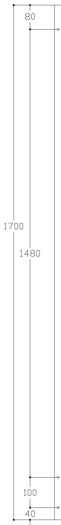
Plan face 2 ( coté opposé ) tube inox longueur 1.70m Percement diamètre 6mm
