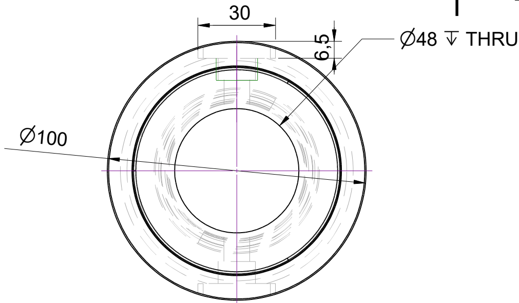
Ferrule CLAMP DIN DN50
