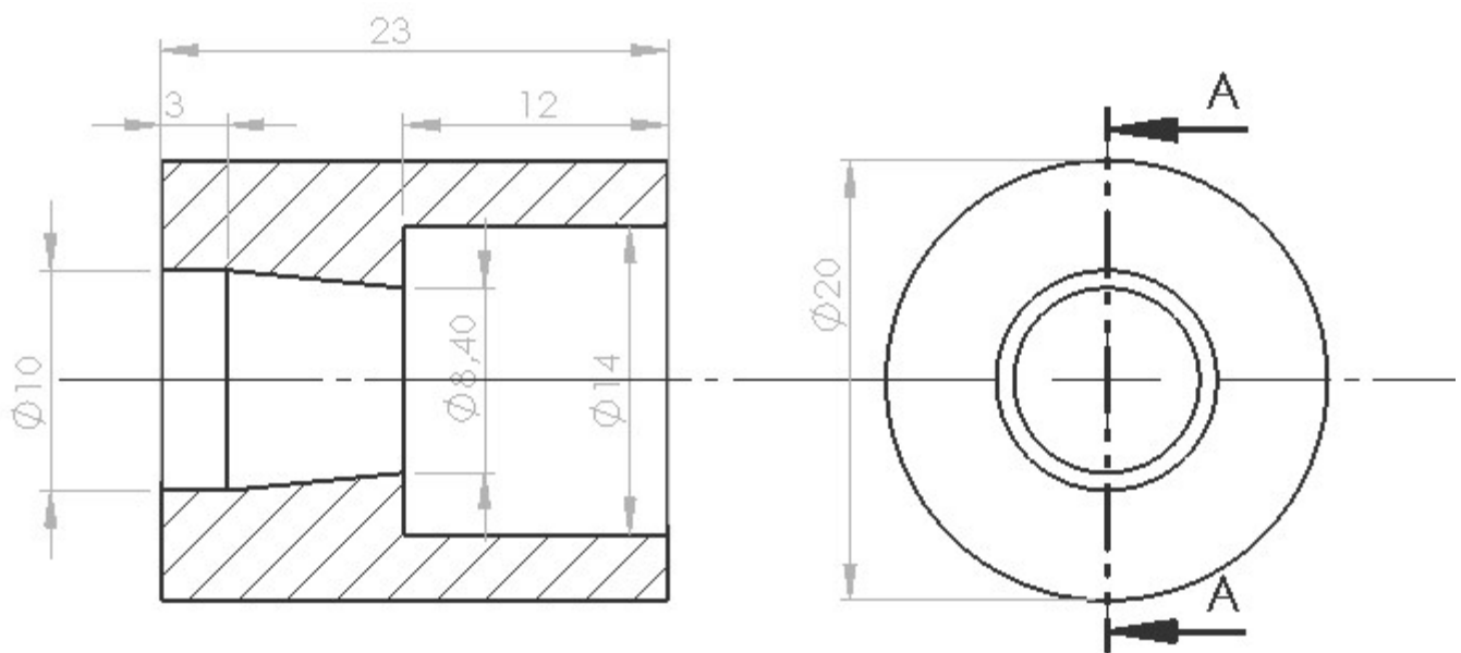
COUPE A-A
