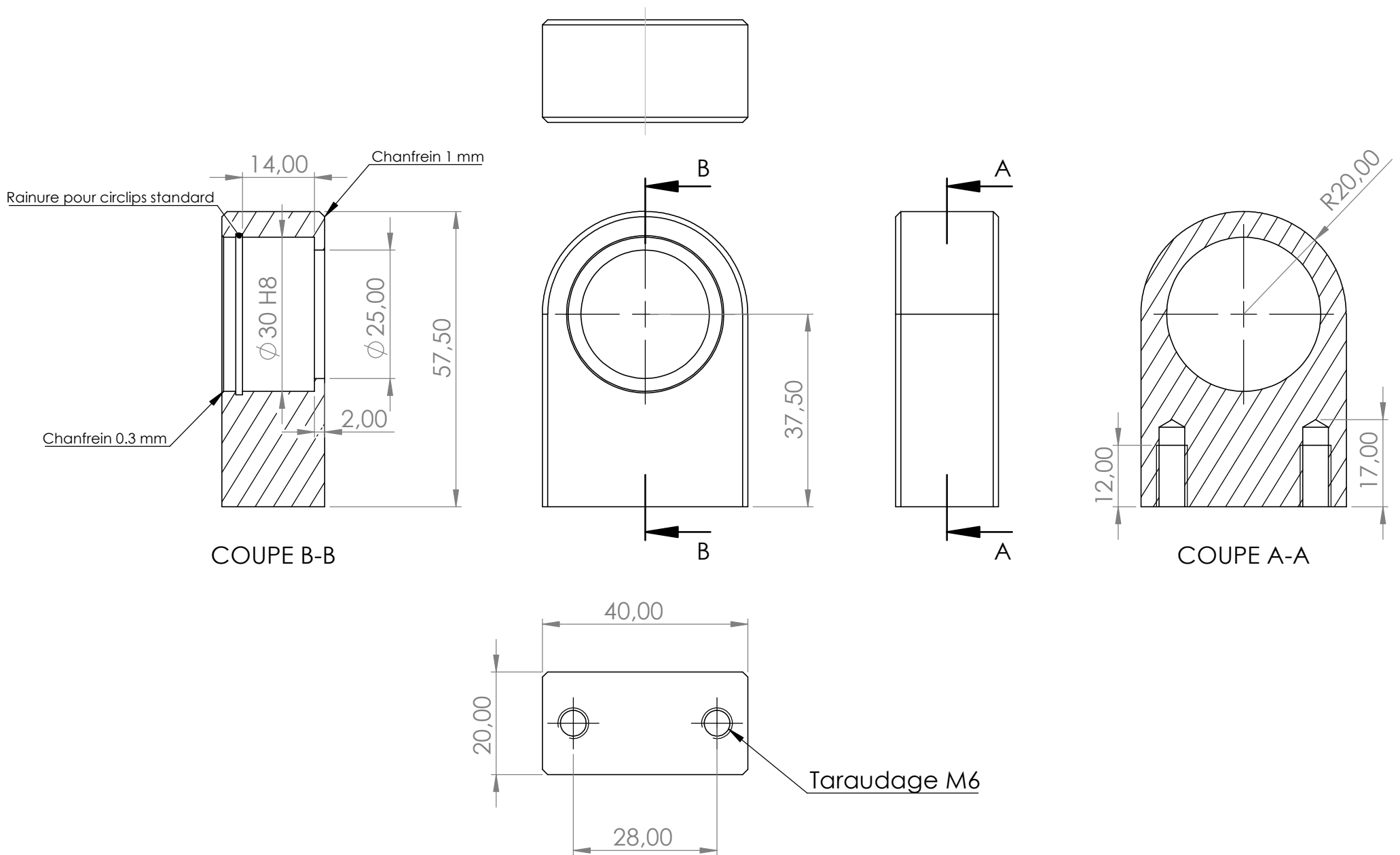
Tête porte roulement Echelle 1:1
