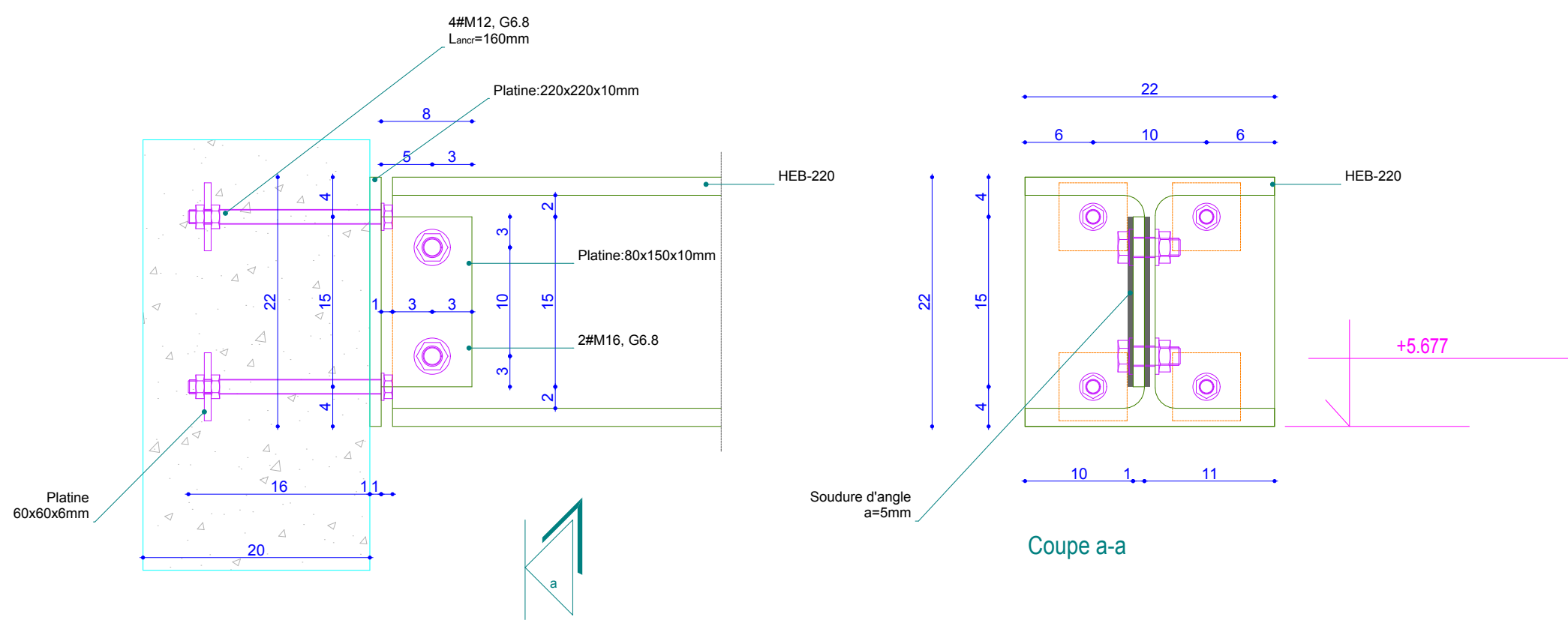
DETAIL 01: PLATINES DE FIXATION HEB - PH RDC
