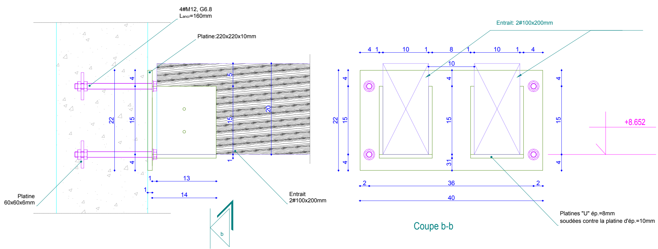
DETAIL 02: PLATINES DE FIXATION ENTRAIT DOUBLE - PH R+1
