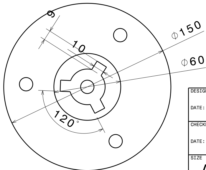
Vue de face Echelle : 1:2
