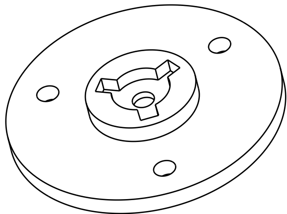
Vue isométrique Echelle : 1:2
