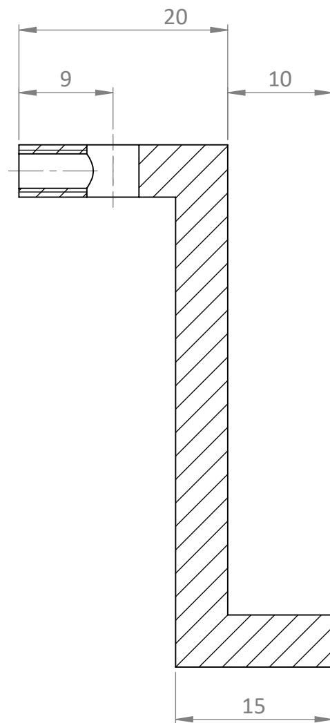
SECTION A-A
