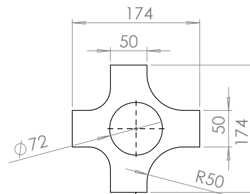
Platine inter Ep 10 S 235 Ech 1/5 Qté 1
