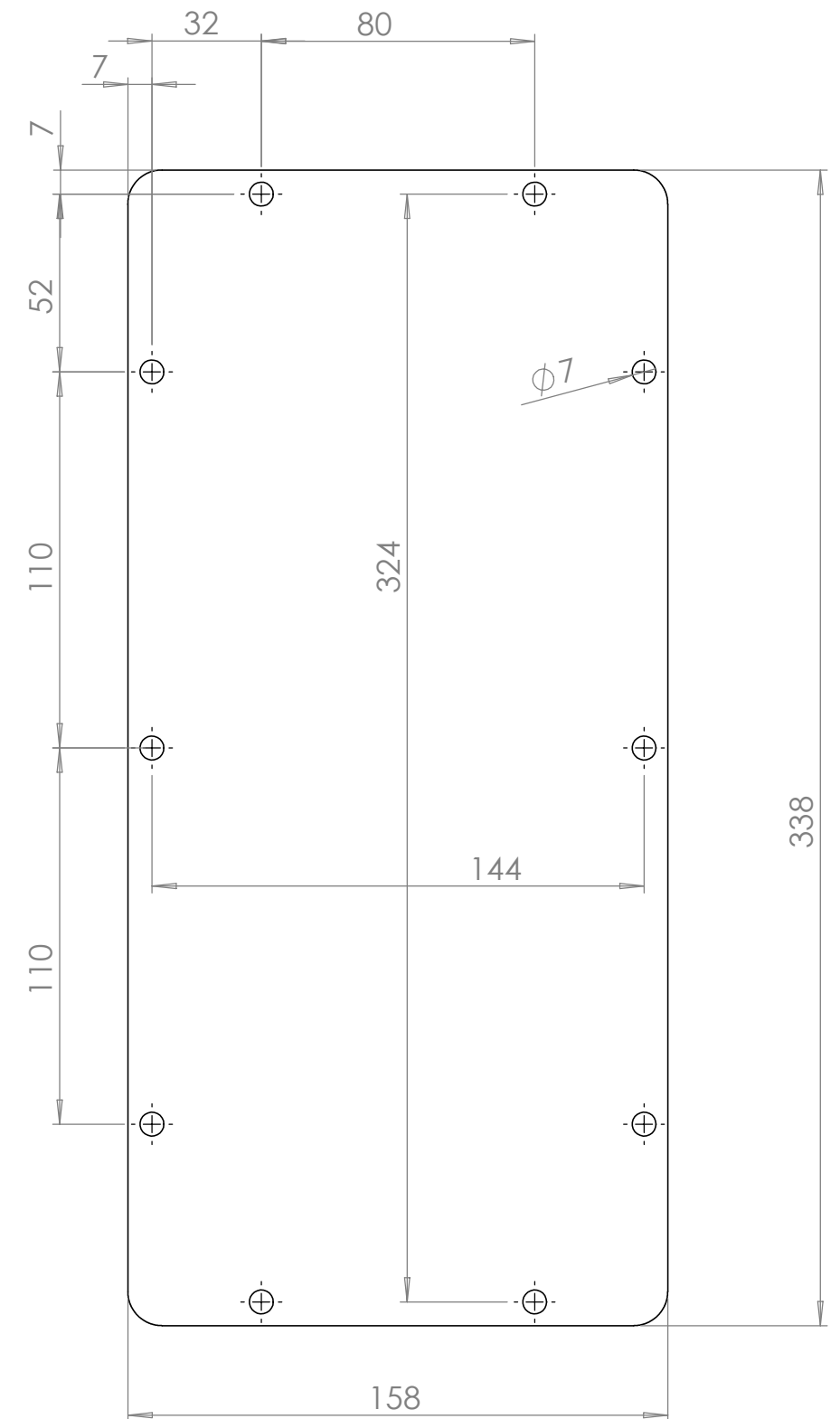
Couvercle S 235 Ep 5 Ech 1/2 Qté 1
