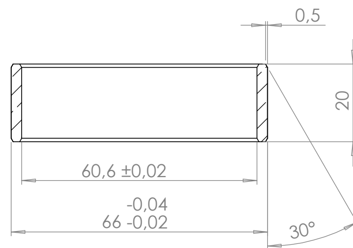
Rep 6 Bague sur tubecentral Bronze Ech 1 Qté 2
