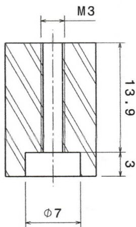
SECTION A-A
