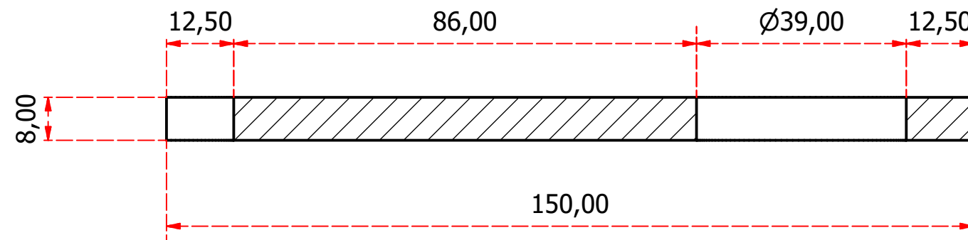
A-A ( 1 : 1 )
