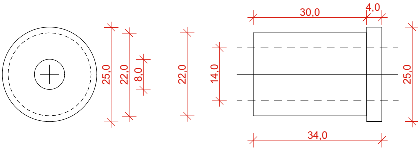
BAGUE ÉPAULÉE EN ACIER CLASSIC SANS TARAUDAGE
