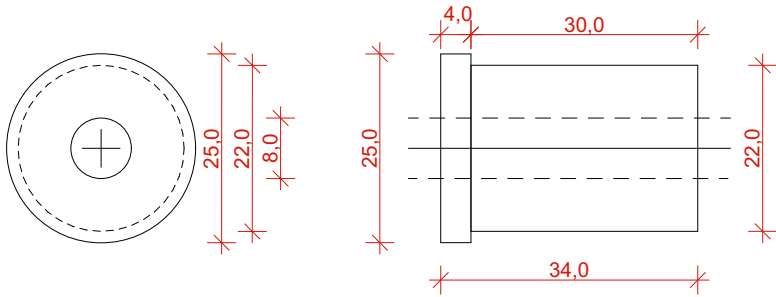
BAGUE EPAULÉE EN ACIER À TARAUDÉS DE PART EN PART POUR RECEVOIR UNE VIS BTR DE 8MM
