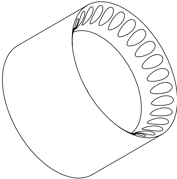
28 perçages diamètre 5mm
