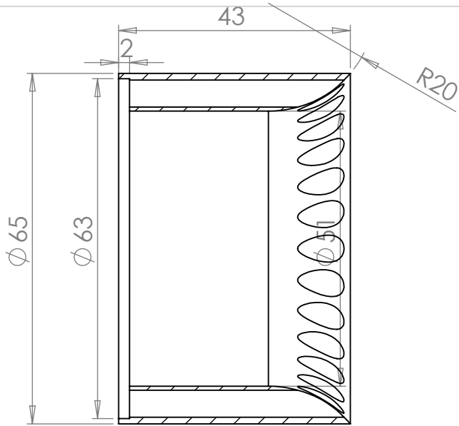
COUPE C-C
