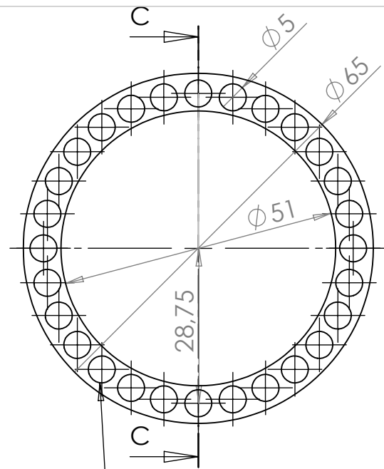
28 perçages diamètre 5mm
