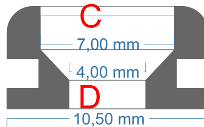
Profil longitudinal (vue au bord de la pièce)
