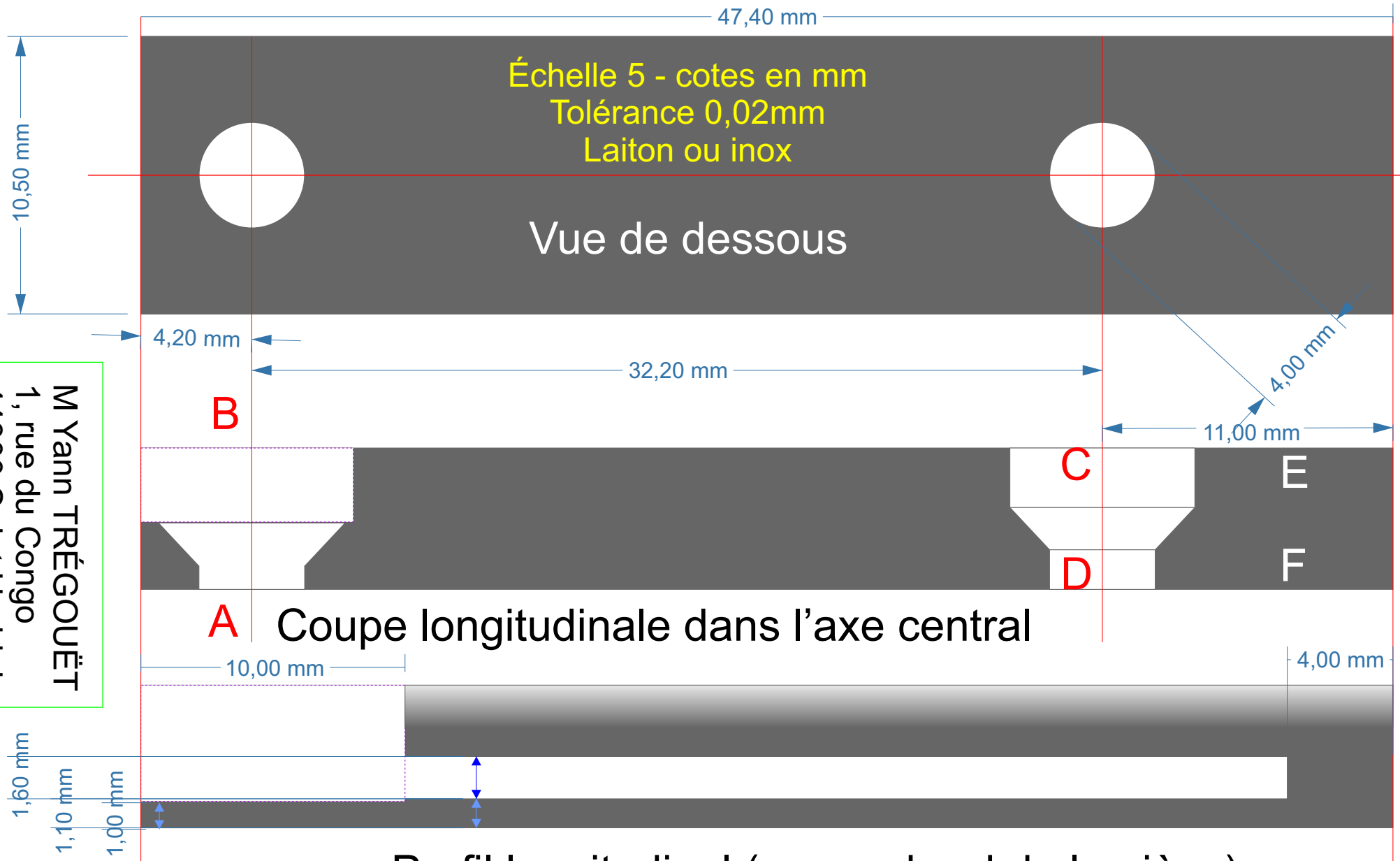
Profil longitudinal (vue au bord de la pièce)
