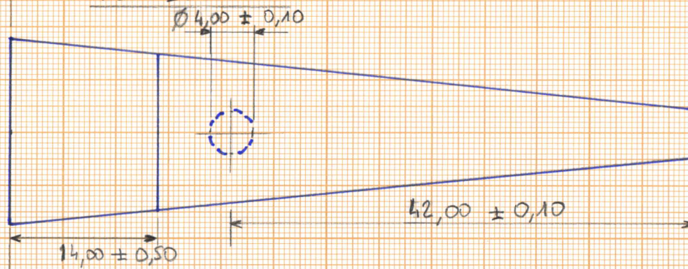
VUE DESSOUS
