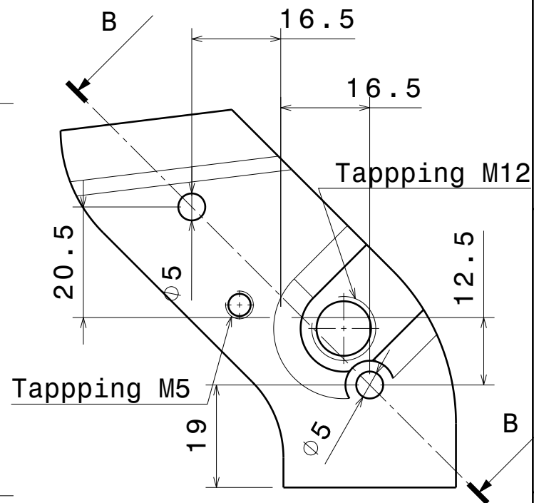
Vue de droite Echelle : 1:1
