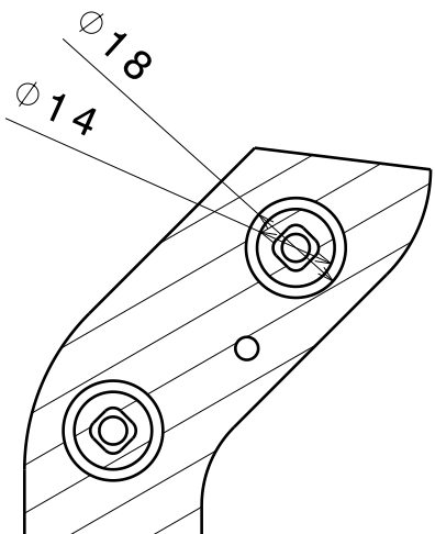
Coupe C-C Echelle : 2:3
