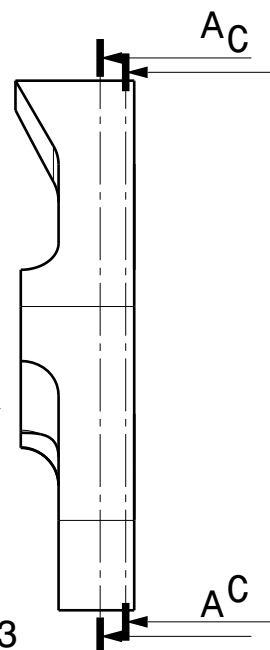
Vue de droite Echelle : 1:1
