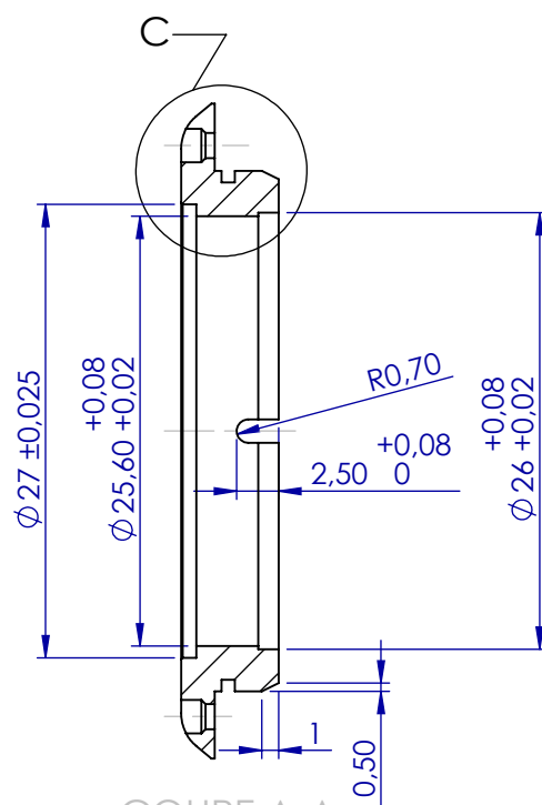
COUPE A-A
