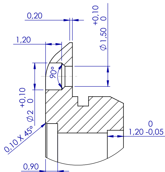
DÉTAIL C ECHELLE 6 : 1
