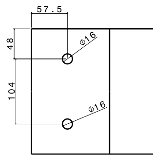
Vue de derrière Echelle : 1:1
