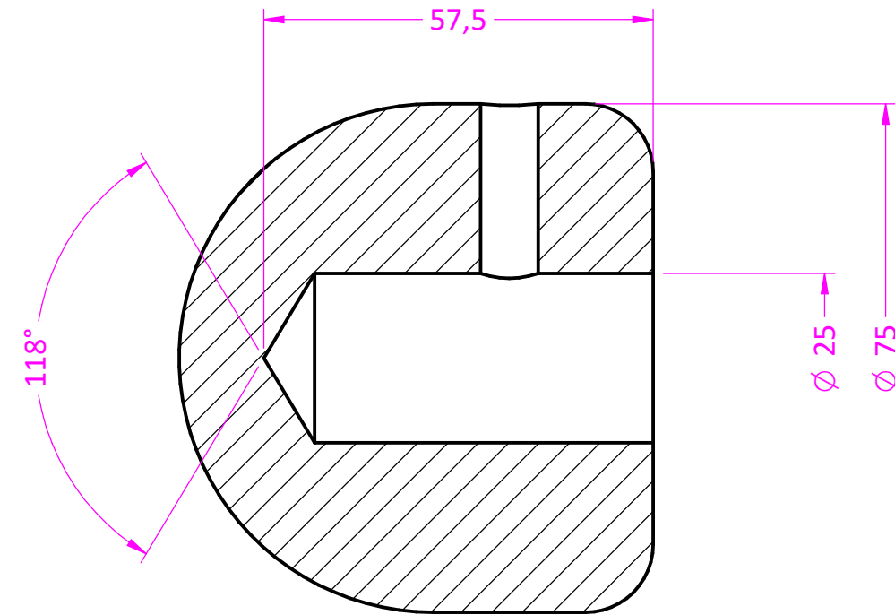
COUPE A-A
