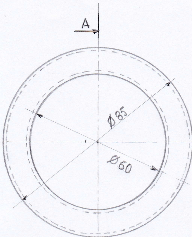
VUE DE DESSUS
