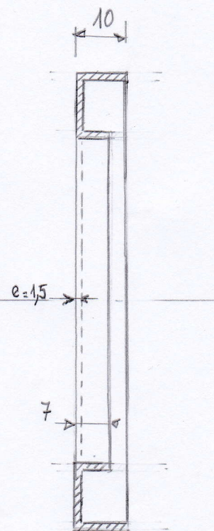
COUPE SUIVANT A-A
