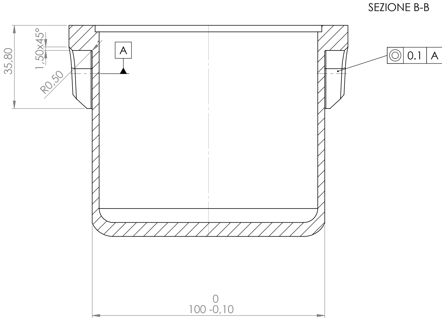
SEZIONE B-B
