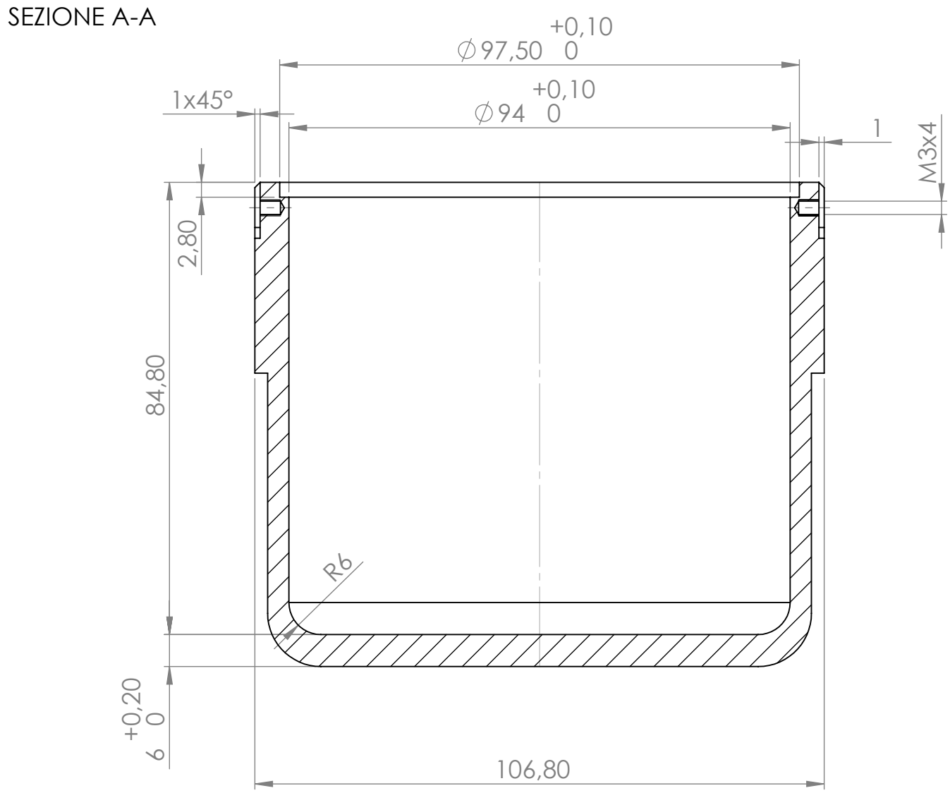
SEZIONE A-A
