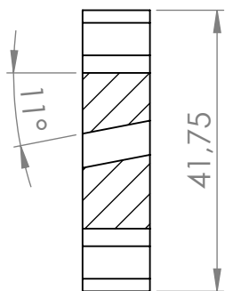
COUPE B-B
