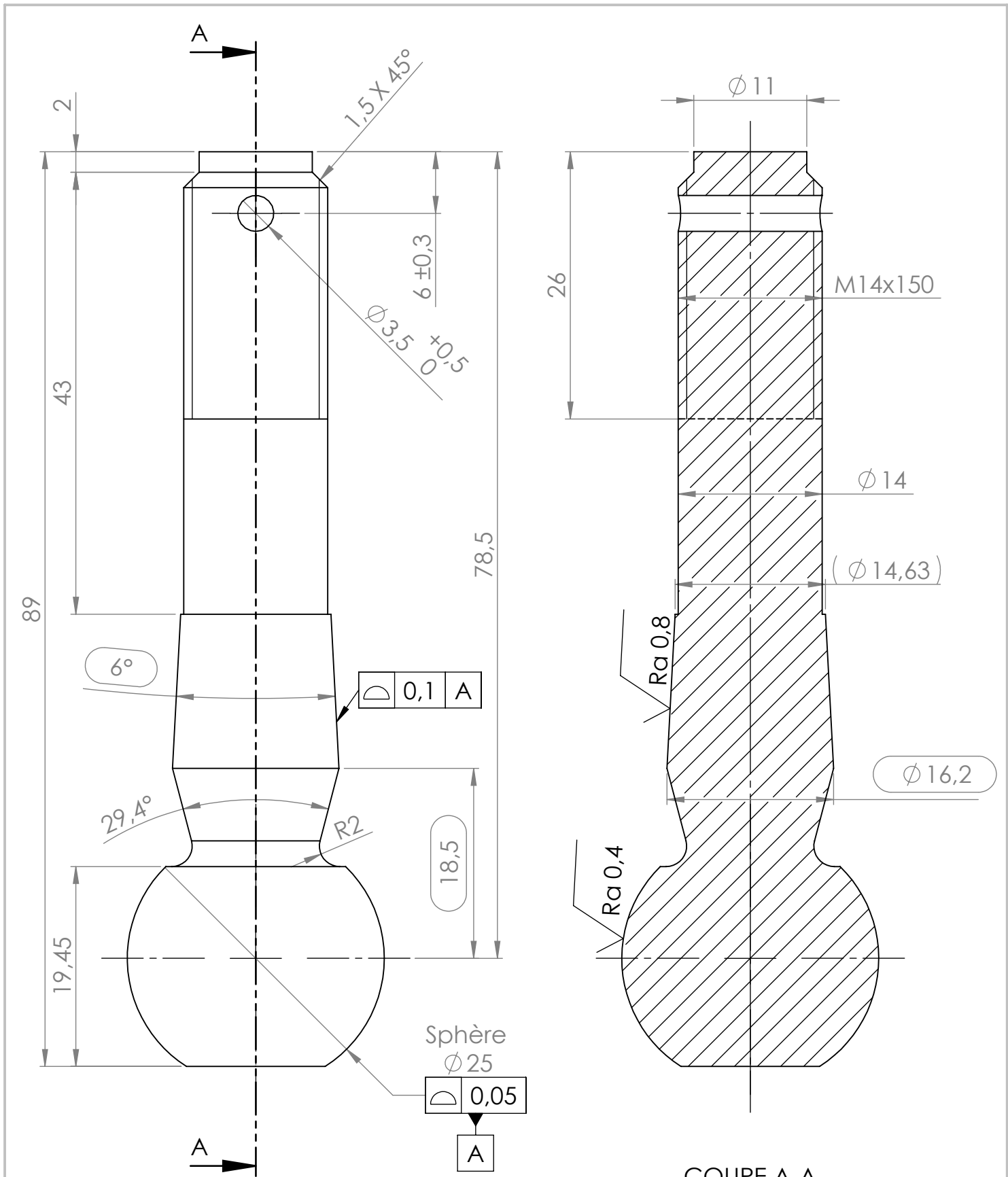
COUPE A-A
